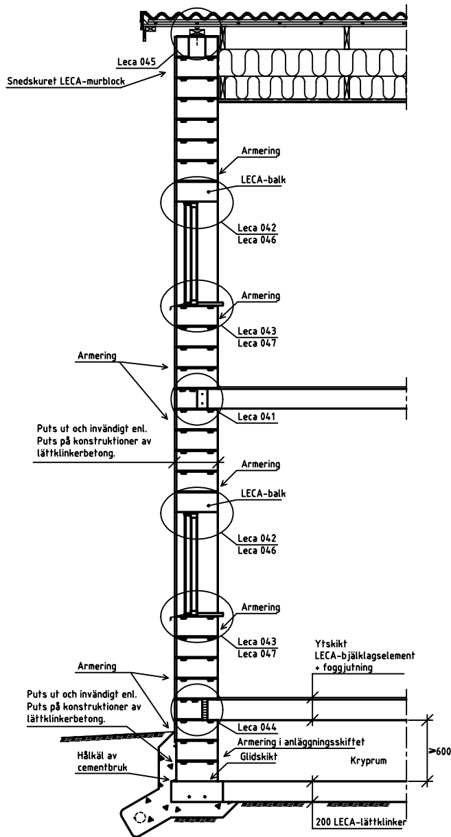
Leca 033 Massiv vägg 1 o 2-plans gavelfasad 1:50
