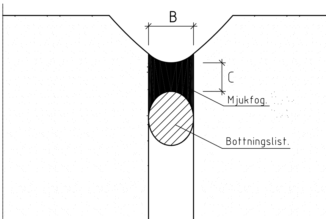
Vertikal rörelsefog.
