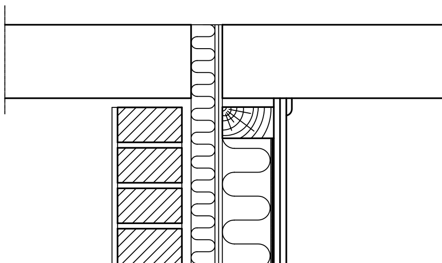
Horisontell rörelsefog vid utstickande byggnadsdel.
